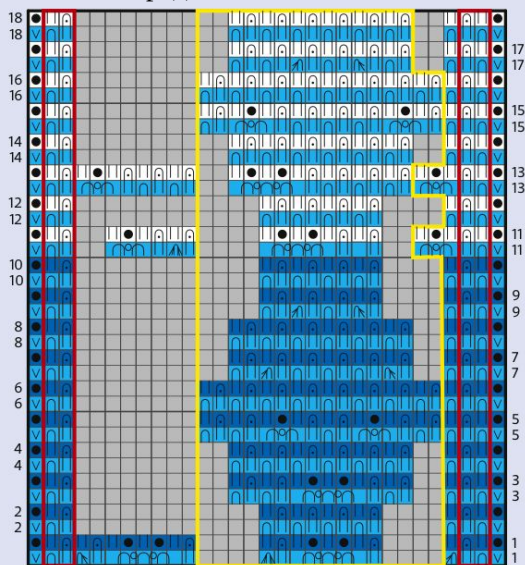
Схема Переда
