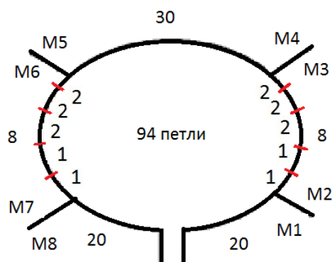
Схема распределения поворотных петель в рукавах
