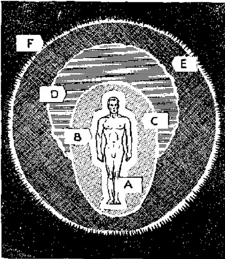
Схема магнитных полей человека
