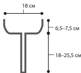
Вырез с вертикальными планками
