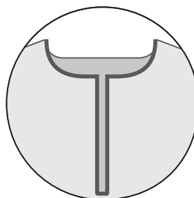
Вырез с вертикальными планками
