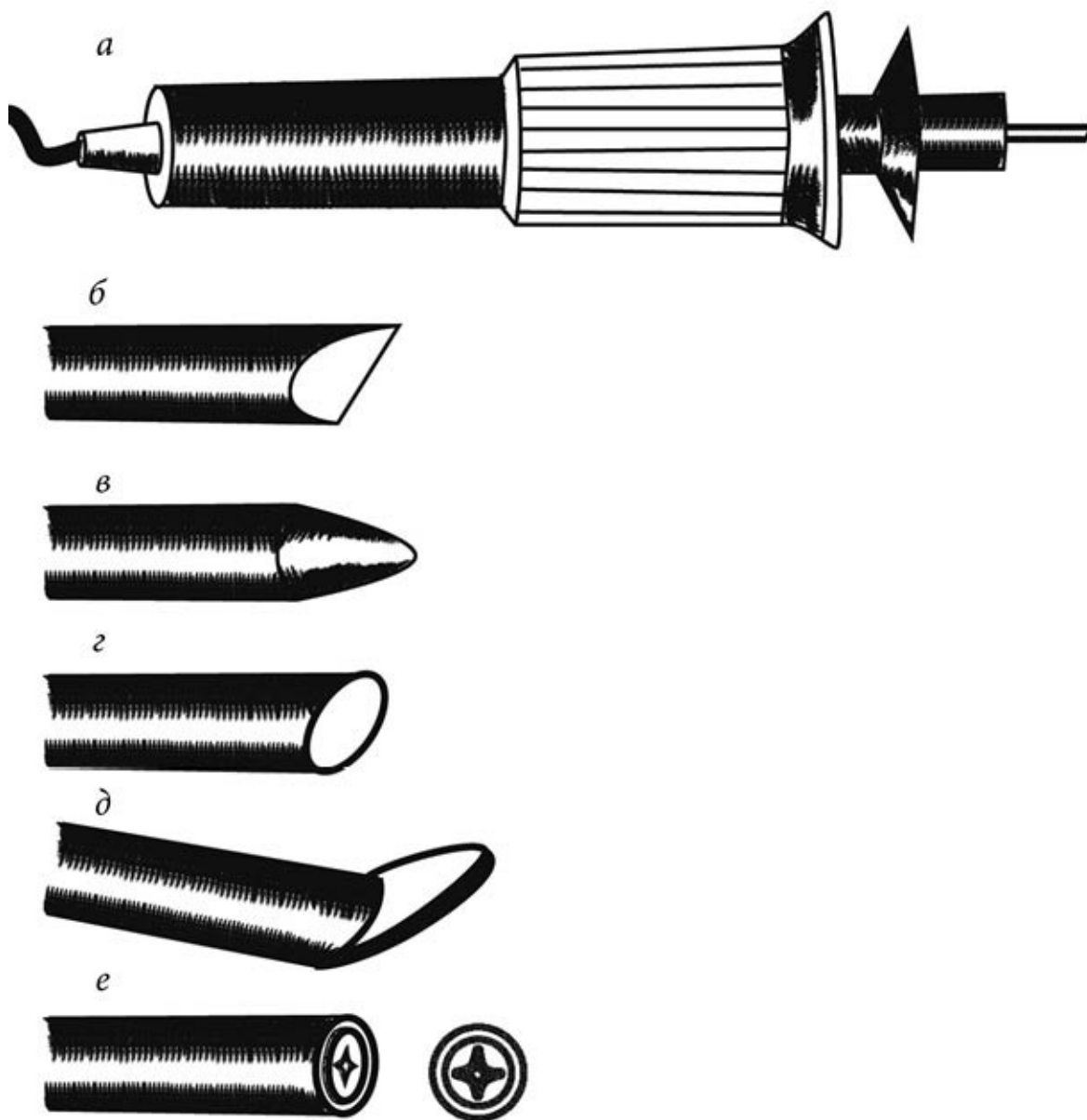
Рис. 4. Пирографический прибор с твердыми насадками: а – пирограф; б – косяя насадка; в – писчая (каллиграфическая) насадка; г – плоский ретушер; д – ложковидный ретушер; е – пример насадки с печатью (штампом)
