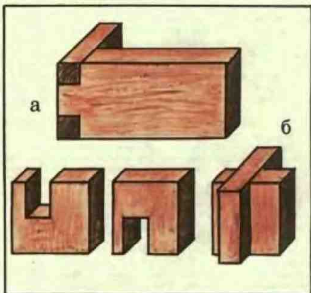
V. Виды соединений: а – в шип; б – в замок
