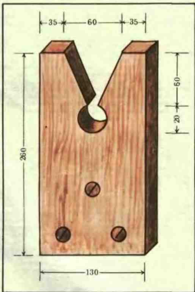
IV. Упорная доска
