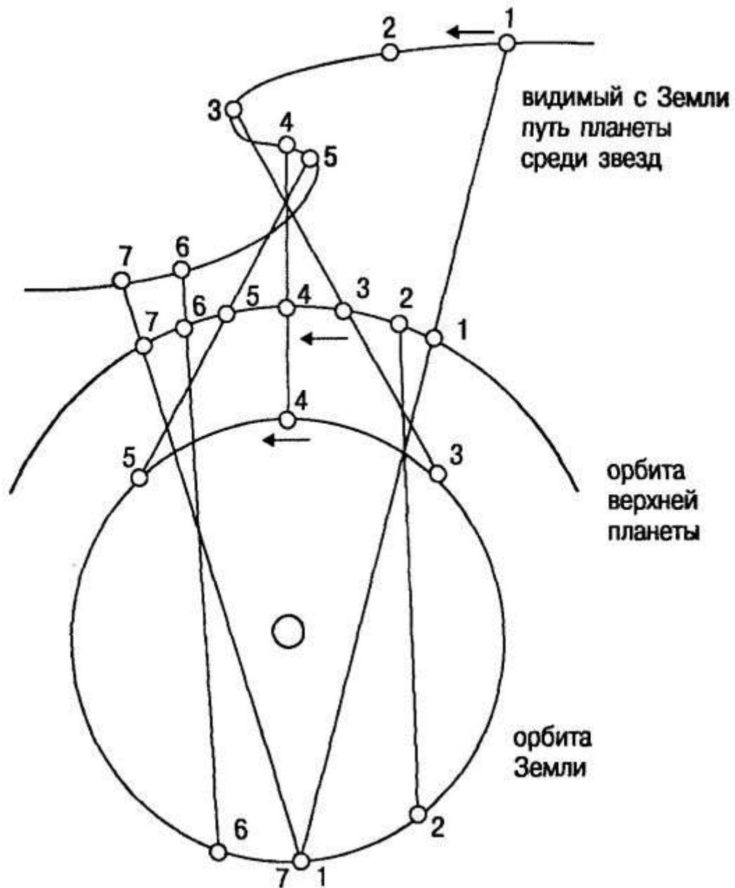
Рис.4.4. Объяснение попятного движения верхних планет
