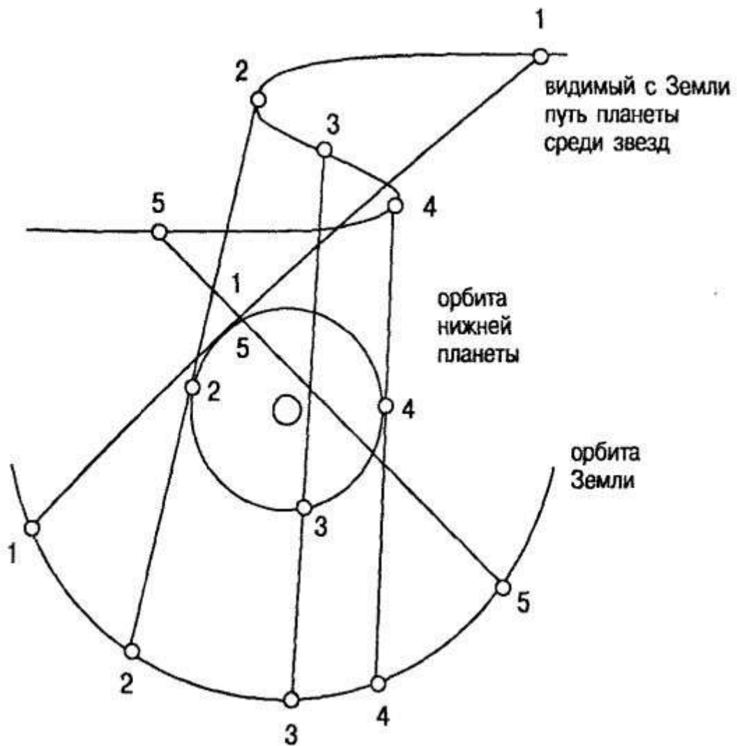
Рис. 4.5. Объяснение попятного движения нижних планет
