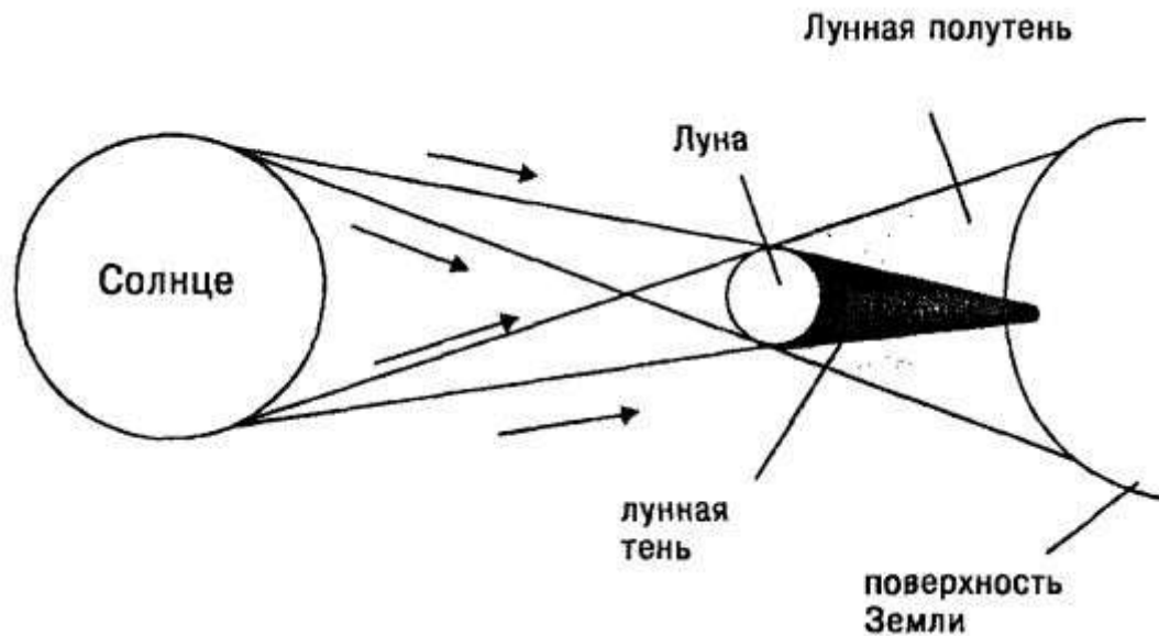
Рис.3.7. Схема солнечного затмения
