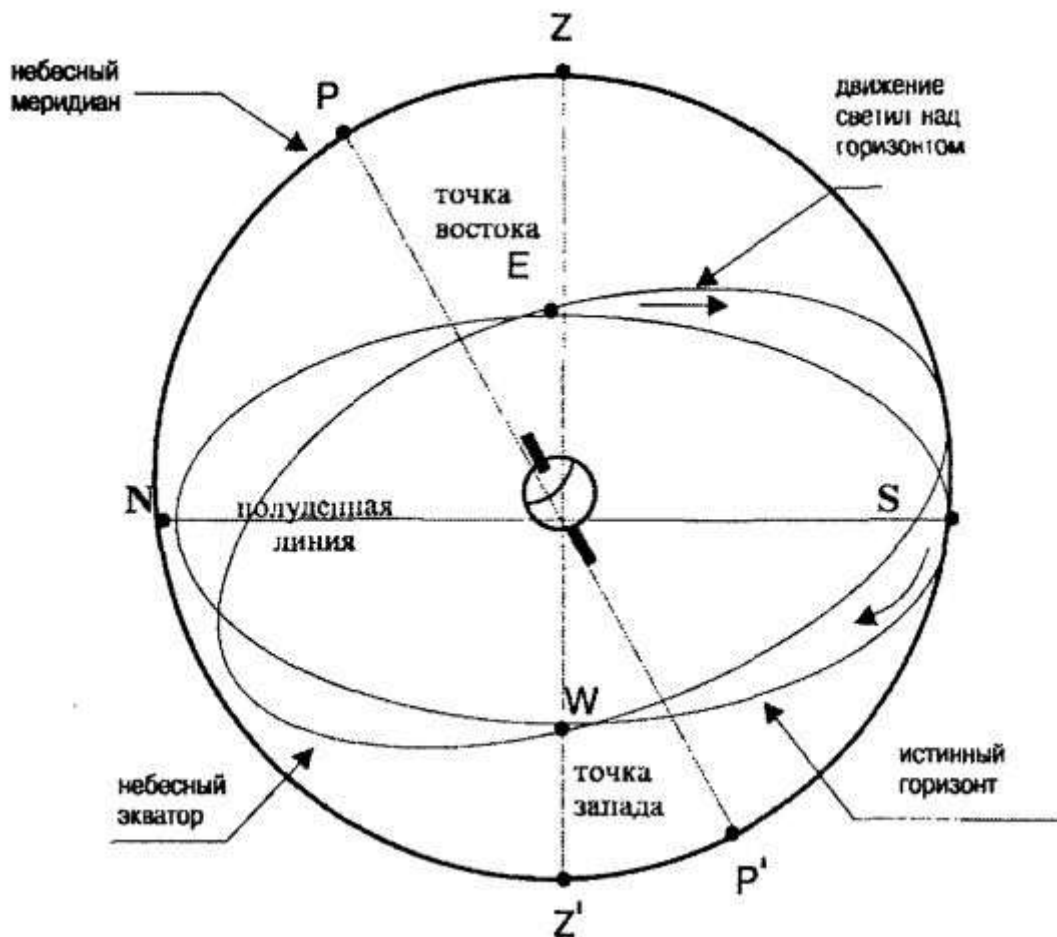
Рис.3.1. Пересечение небесного экватора и небесного меридиана с истинным горизонтом
