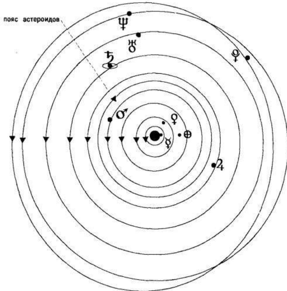
Рис.3.6. Орбиты планет Солнечной системы
