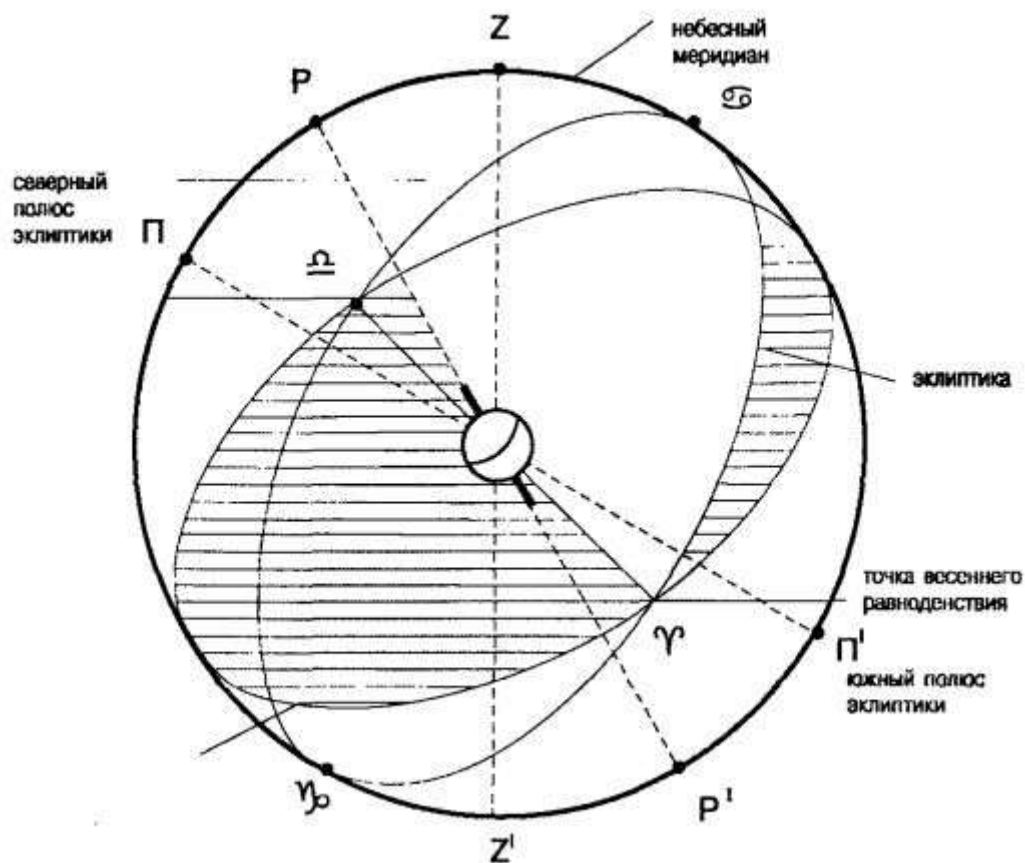
Рис.3.2. Плоскость эклиптики и её пересечение с плоскостью небесного экватора
