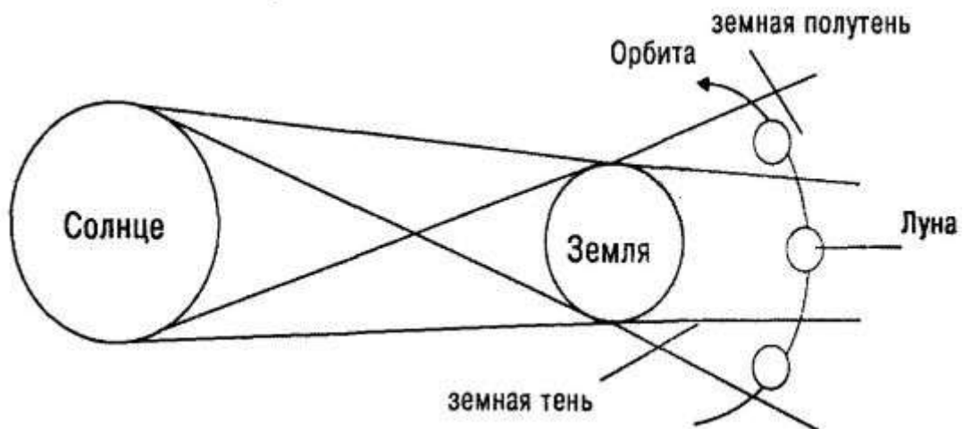
Рис.3.8. Схема лунного затмения
